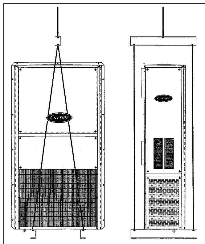
Figura 1 - Içamento
