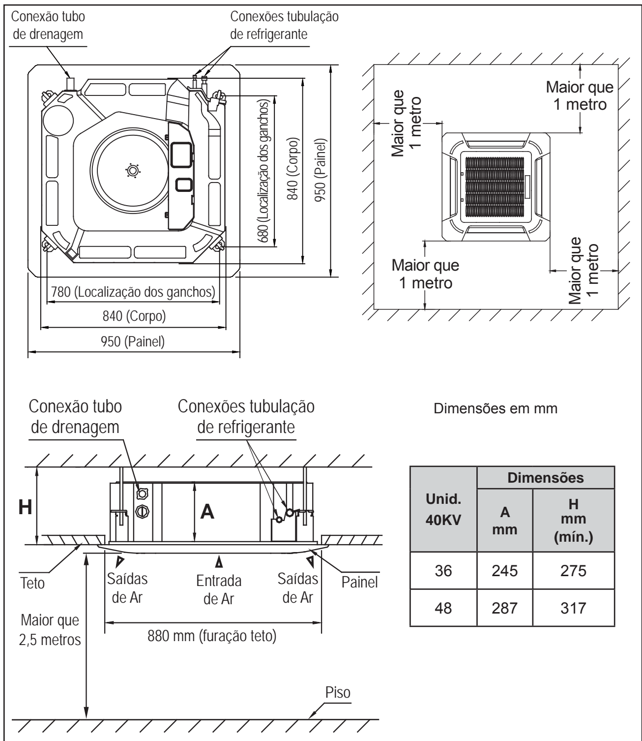
FIG. 9 - DIMENSIONAL E ESPAÇAMENTOS MÍNIMOS
