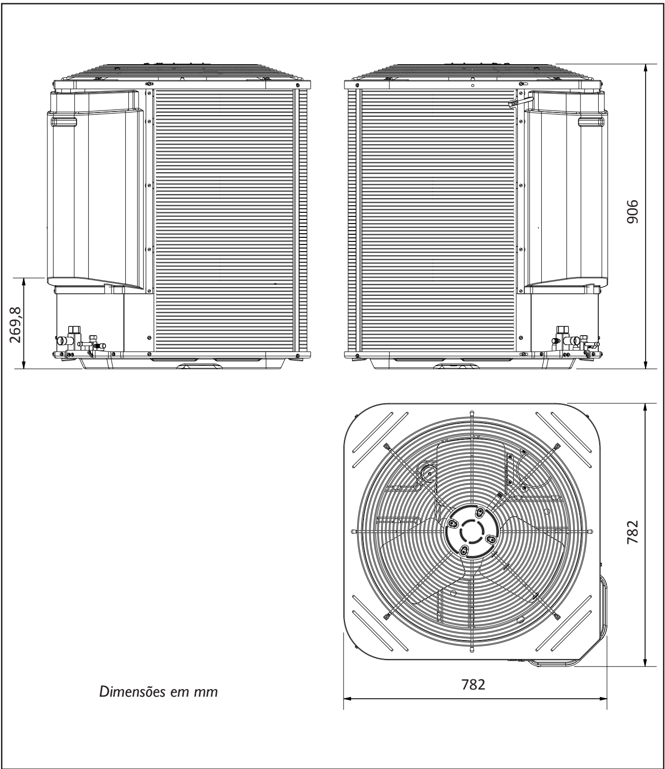
FIG. 7 - DIMENSIONAL UNIDADES CONDENSADORAS 38CCV60
