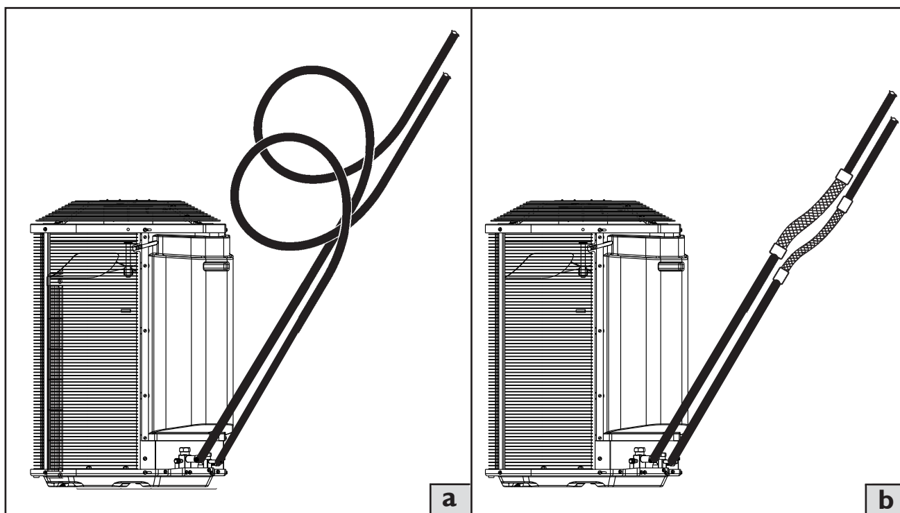
FIG. 35 - INSTALAÇÃO DOS LOOPS
