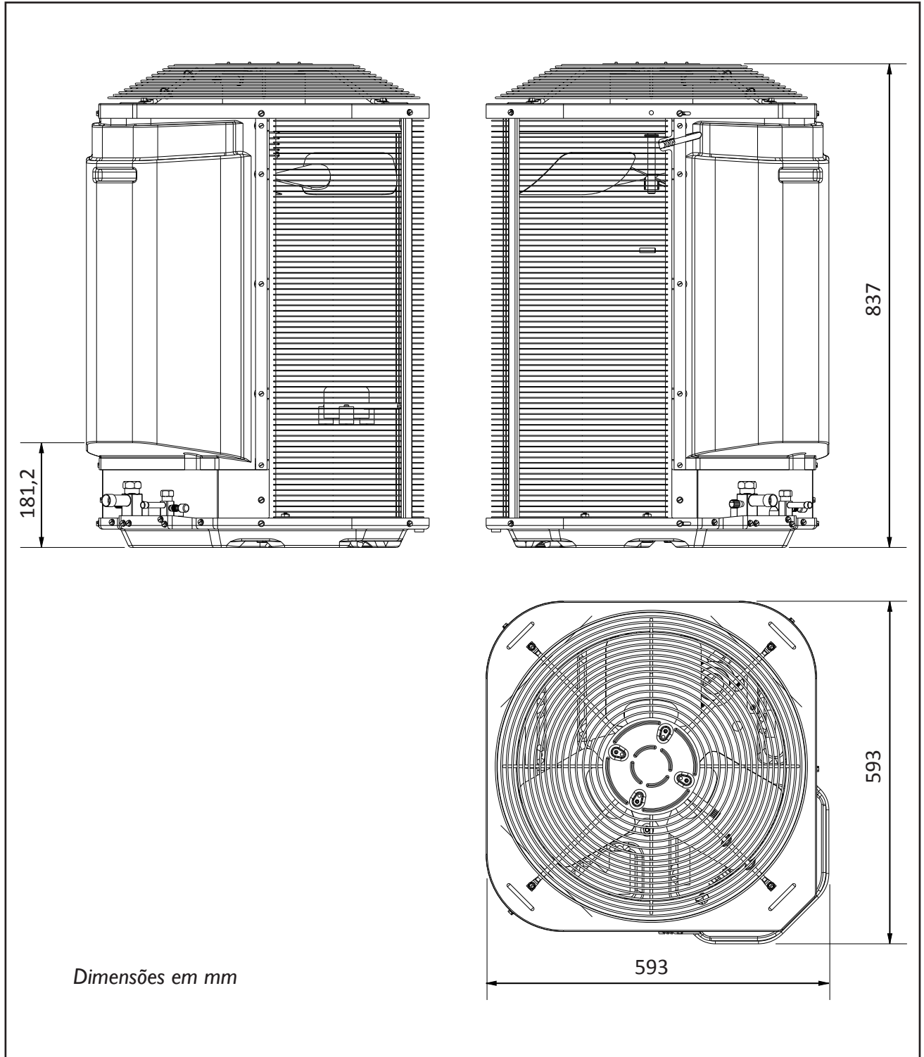
FIG. 6 - DIMENSIONAL UNIDADES CONDENSADORAS 38CCV36
